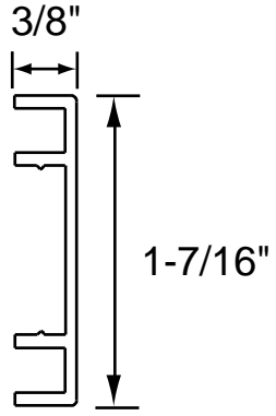
306 Trim
