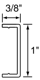
302 Trim
