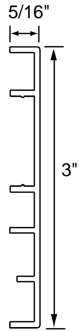
304-3 Trim
