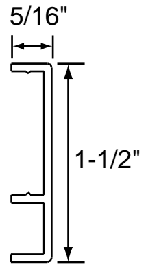
304-1 Trim
